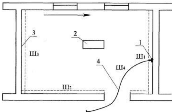
Рис. 27. Схема организации рабочего места звена № 1
