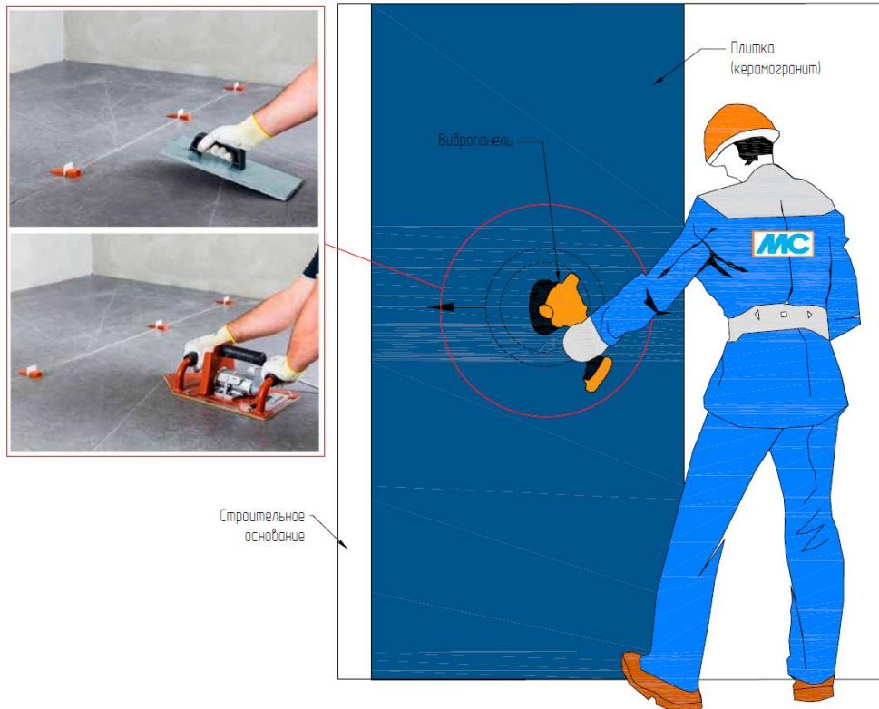
Рис. 39. Увеличение адгезии плитки с основанием вибрированием или простукиванием
