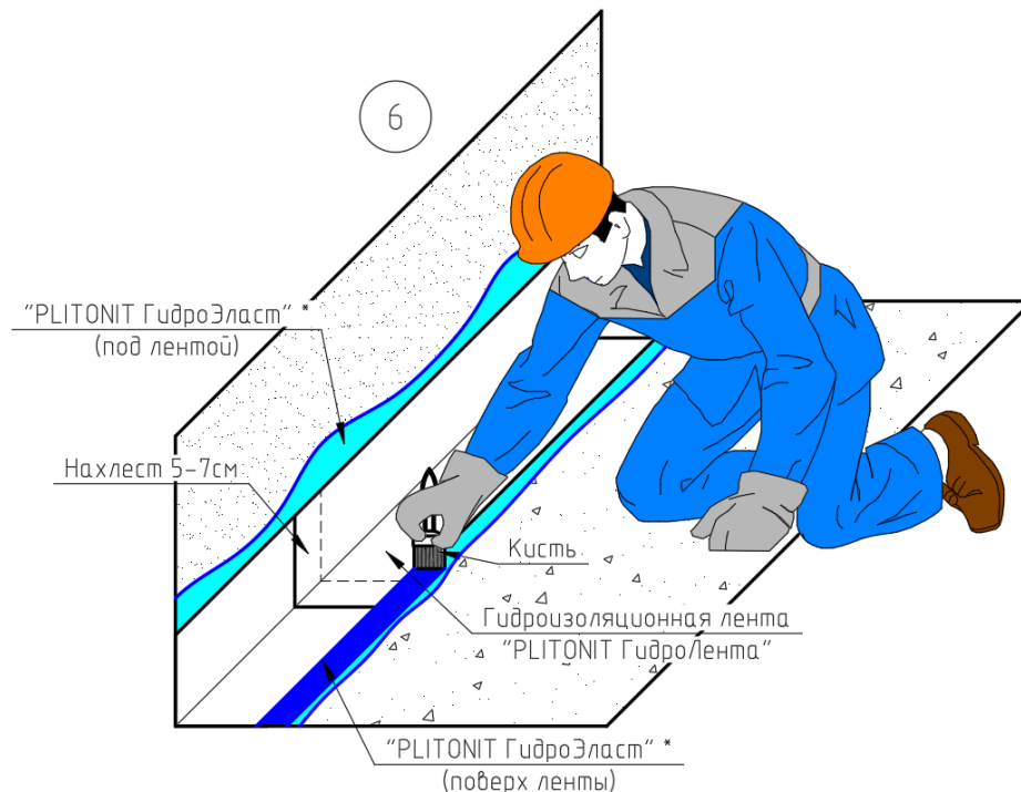
Рис.32. Последовательность работ, где: 1 - проверка ровности основания контрольной рейкой (аналогично для горизонтальной поверхности); 2 – размешивание емкости с мастикой; 3 – нанесение первого слоя мастики, разбавленной водой в пропорции 1:10, на основание; 4 – нанесение гидроизоляции на поверхность (аналогично для горизонтальной поверхности); 5 – укладка гидроизоляционной ленты на поверхность, предварительно обработанную «PLITONIT ГидроЭласт» или «PLITONIT WaterProof Standard»; 6 – поверхностная обработка ленты мастикой «PLITONIT ГидроЭласт» или «PLITONIT WaterProof Standard».
