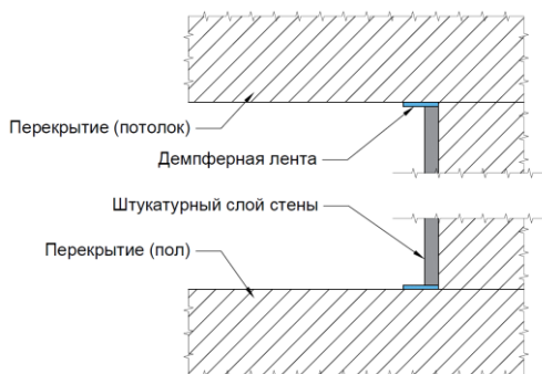
Рис.25. Приклейка демпферной ленты в местах сопряжения штукатурного слоя со стеной и потолком
