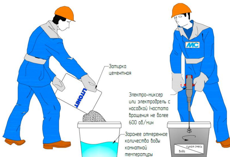
Рис. 42. Приготовление состава
