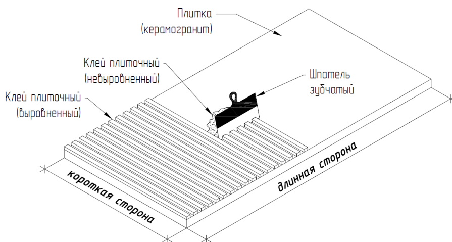
Рис. 33. Нанесение плиточного клея на плиту
