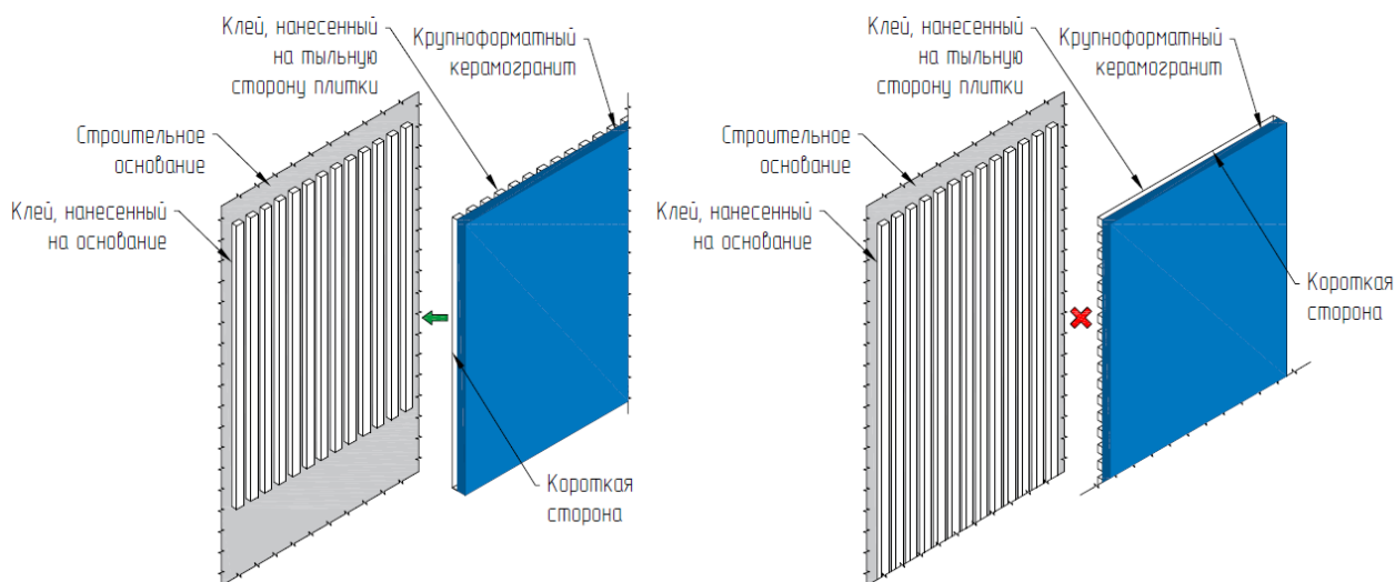
Рис. 34. Клей следует наносить в одном направлении на основание и на плитку
