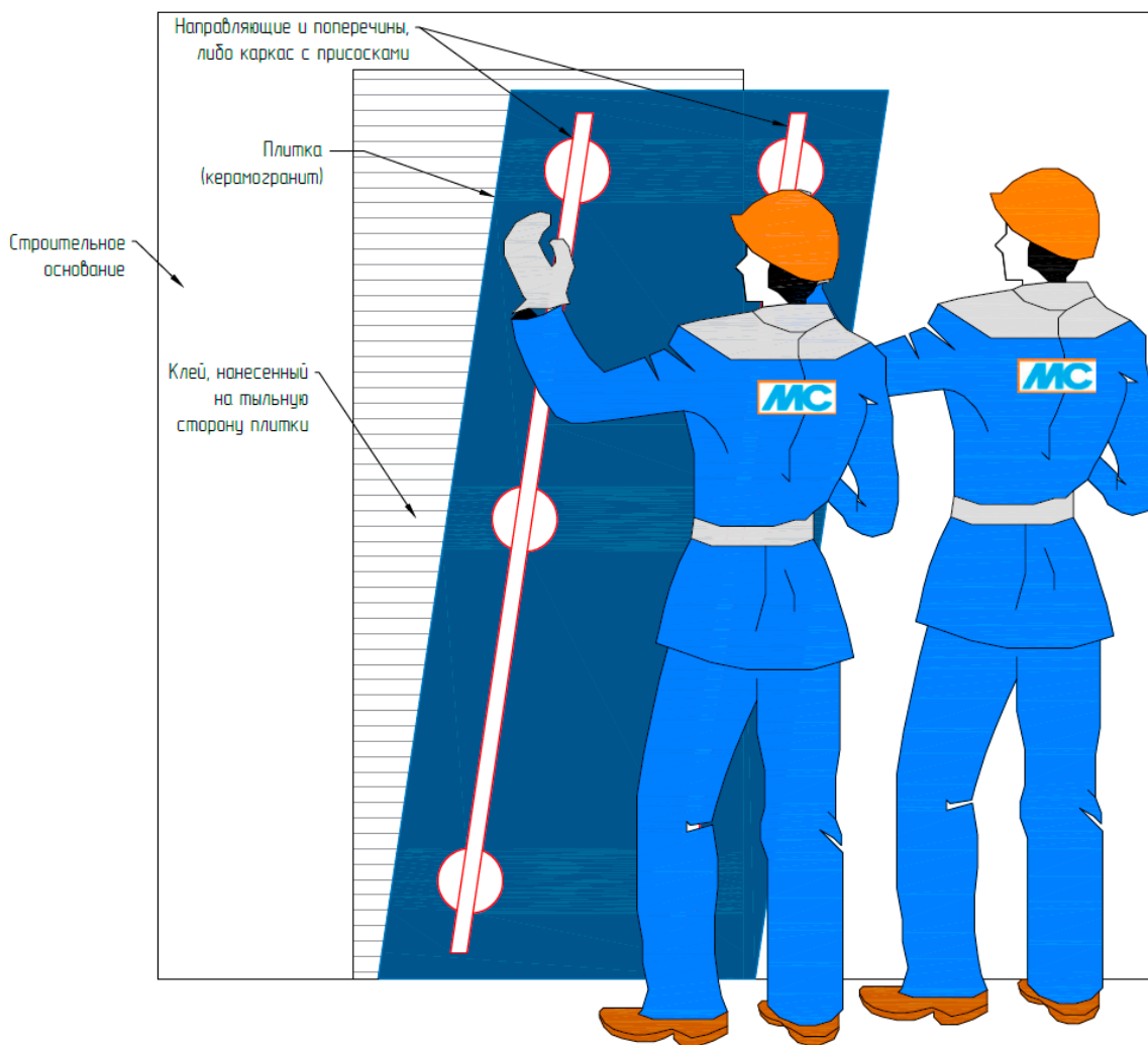
Рис. 38. Монтаж крупноформатного керамогранита
